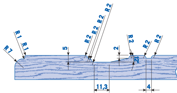
Profilo/Profile/Profil/Profil/Perfil B
